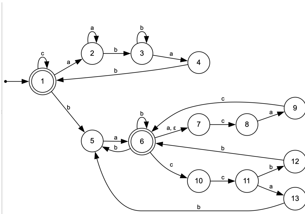
Рис. 2: Граф НКА
