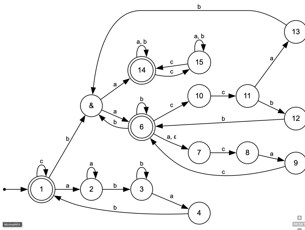
Рис. 3: Граф ПКА
